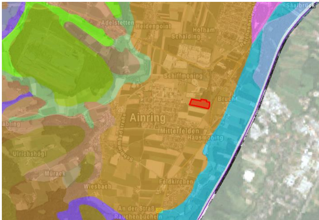
Übersichtsbodenkarte ROT: Lage Plangebiet (BayernAtlas 2023, nicht maßstäblich)
