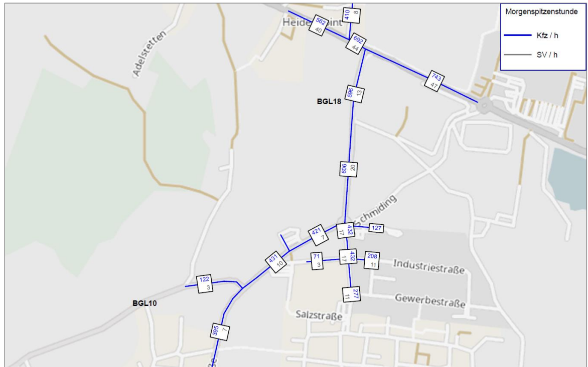
Abbildung 4: Verkehrsmengengerüst werktags Morgenspitze Analyse (Kfz/h und SV/h) – Detail Nord
