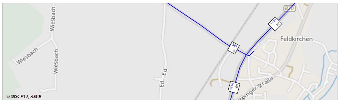
Abbildung 5: Verkehrsmengengerüst werktags Morgenspitze Analyse (Kfz/h und SV/h) – Detail Süd
