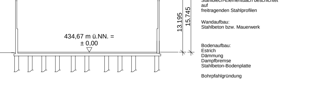
SYSTEMGEBÄUDEQUERSCHNITT M 1:500
