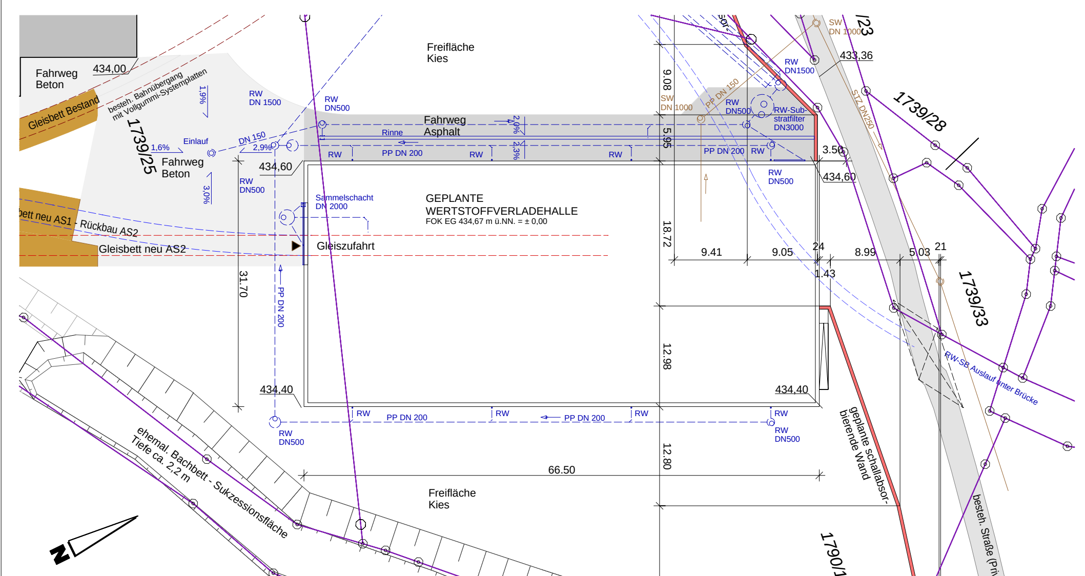
WERTSTOFFVERLADEHALLE GRUNDRISS ERDGESCHOSS M 1:500
